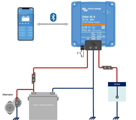
Configuration de connexion typique en tant qu'alimentation CC-CC
