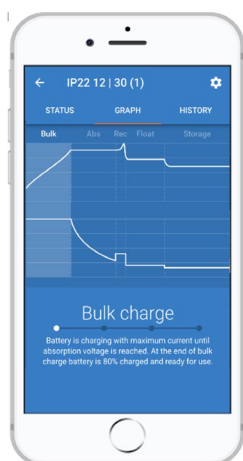
Écran graphique
